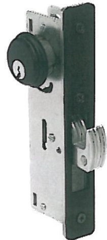
Hook Bolt Mortise Lockset 1-1/8" Duro LH
